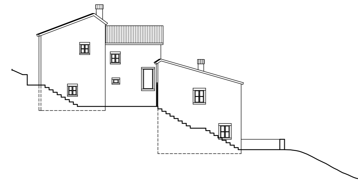
PROSPETTO NORD
