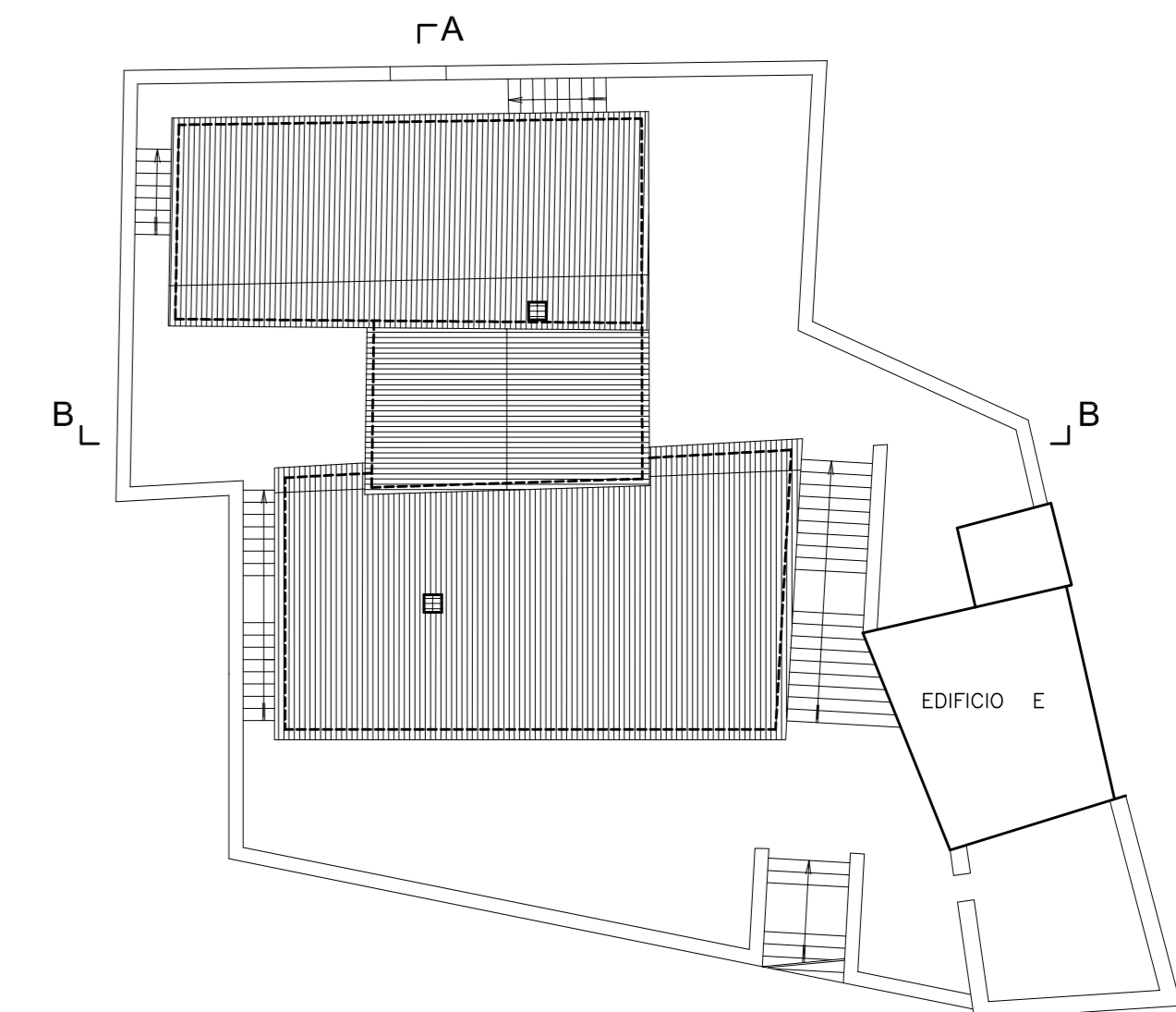
PIANTA PIANO COPERTURA
