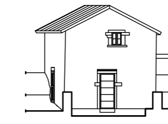
PROSPETTO OVEST
