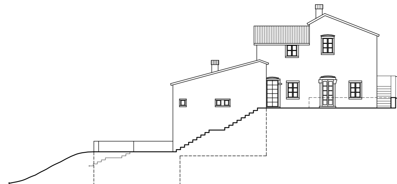
PROSPETTO SUD
